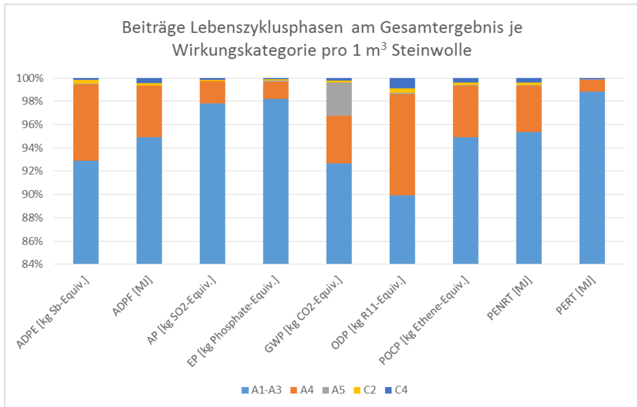
Abbildung 6-1: Ökobilanzergebnisse 1 m 3 Steinwolle
