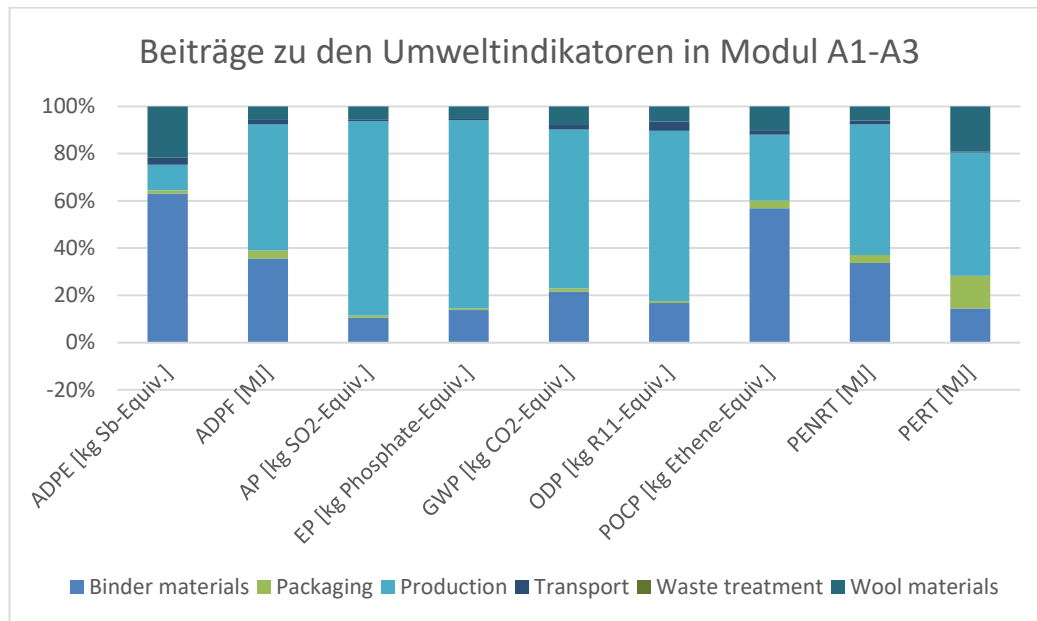
Abbildung 6-2: Dominanzanalyse Modul A1-A3 Steinwolle
